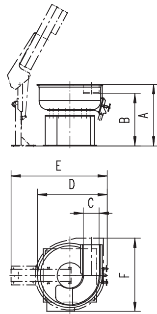
CD Rundvibrator mit Schalldämmdeckel
